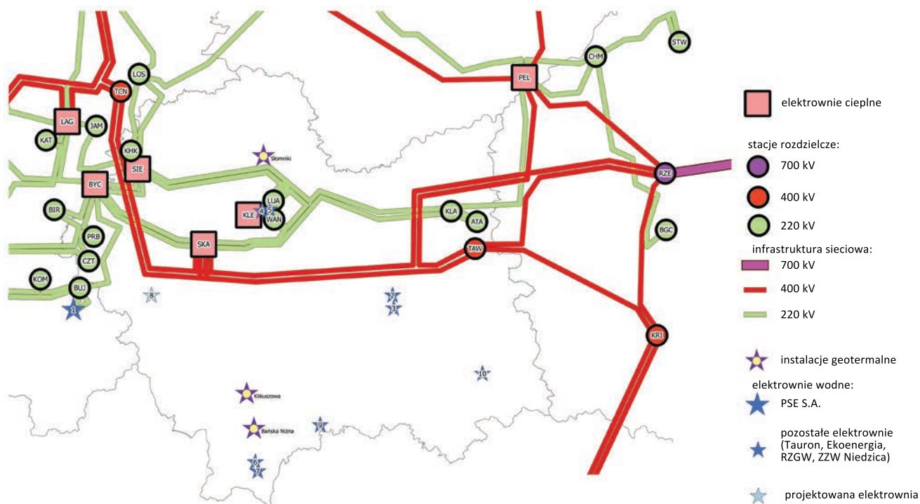
Ryc. 40 System energetyczny w Małopolsce
