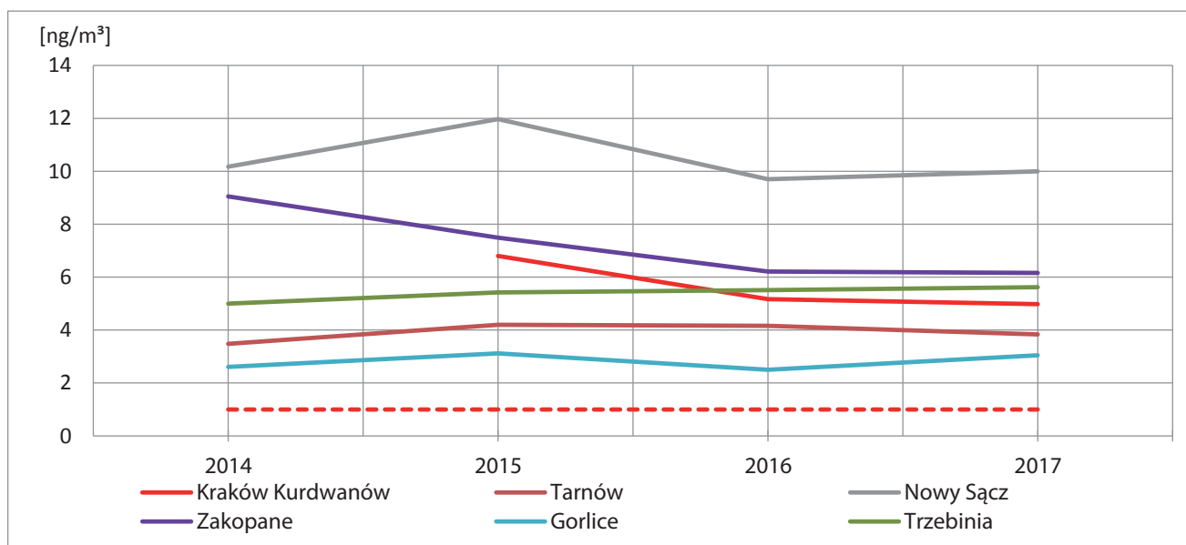
Ryc. 28 Poziom zanieczyszczeń benzo(a)pirenem B(a)P [ng/m 3 ]
