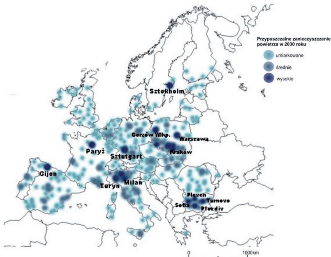
Ryc. 32 Prognoza ostrzegawcza
