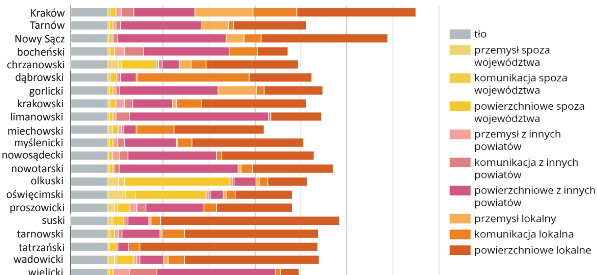
Ryc. 27 Wpływ źródeł emisji na stężenia pyłu PM 2,5 na obszarach przekroczeń poziomu średniorocznego
